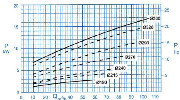
دور موتور ۱۴۵۰ / 1450 rpm
